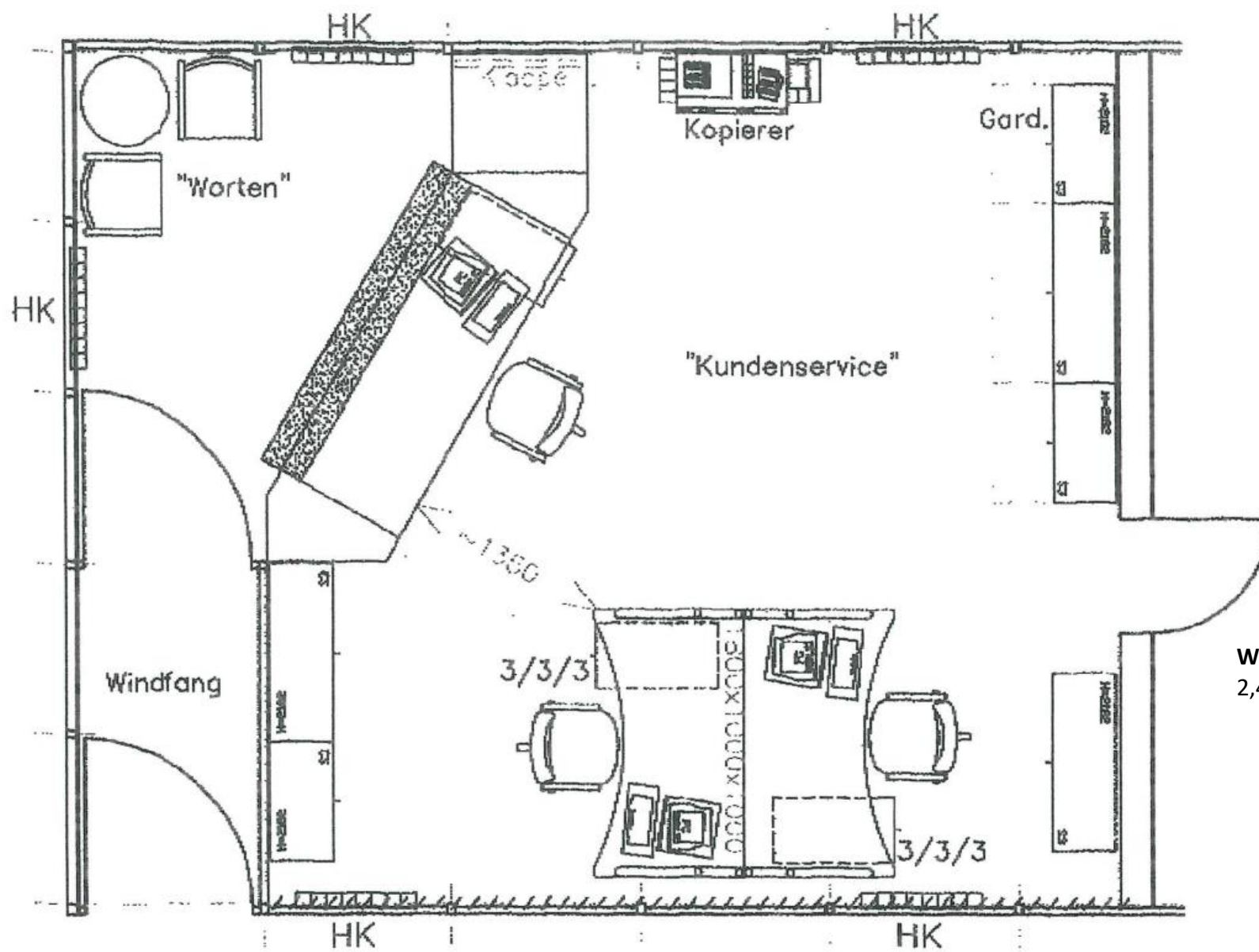
Kundenbüro: 6,50 m x 5,70 m
